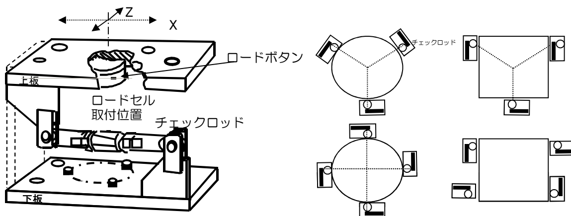
図1、フレックスロック取付け例
