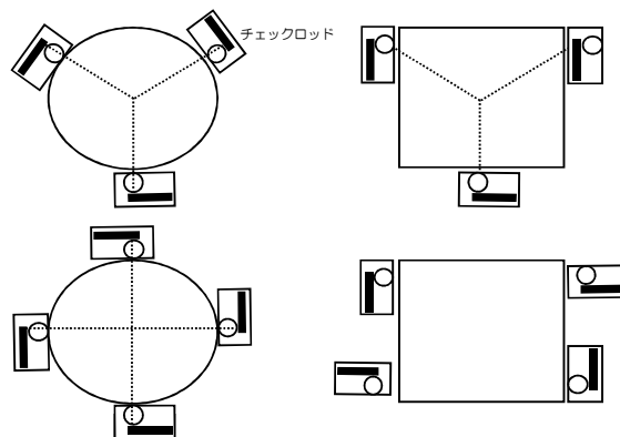
図1, フレックスロック取付け例
